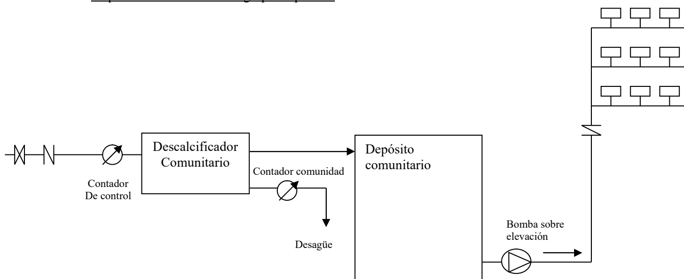
Esquema 2: instalación con grupo de presión
